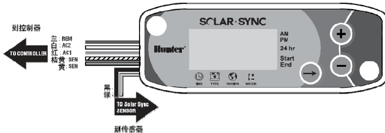
Solar Sync 气候传感器控制器模块导线联接图
